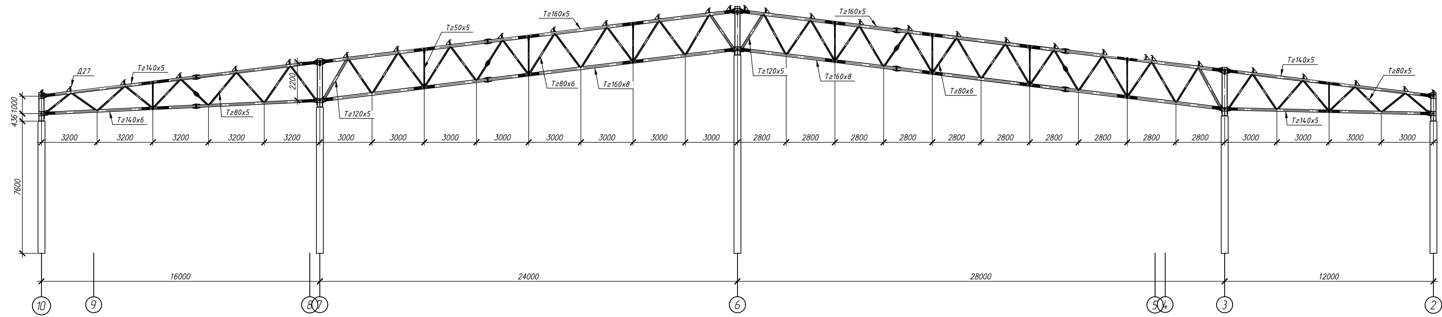
Разрѣз по оси Е
